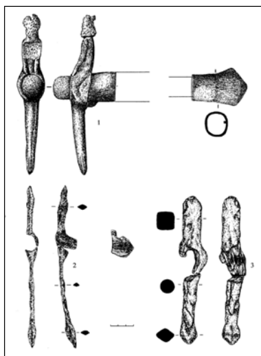
Рис. 5. Чеканы каменной культуры: 1 – Новотроицкое-2, к. 15, м. 3 (по: Шульга, Уманский, Могильников, 2009); 2 – Новотроицкое-1, к. 2, м. 1; 3 – Екатериновка-2, к. 2, м.1. 1–3 – железо
